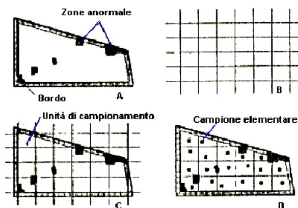
Fig. 2 Campionamento sistematico
